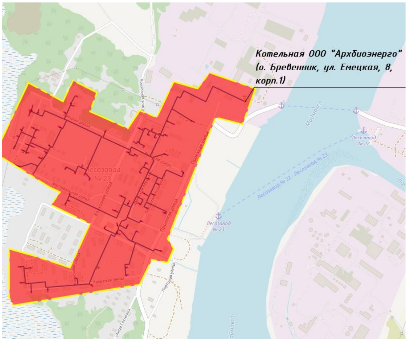
Рисунок 8. Зона действия котельной ООО «Архбиоэнерго» о. Бревенник, ул. Емецкая 8, корп.1
